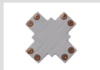
X 字型基盤 3528 品番：HBC3528PCX 5050 品番：HBC5050PCX
