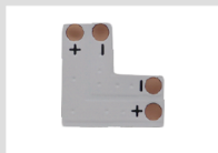
L 字型基盤 3528 品番：HBC3528PCL 5050 品番：HBC5050PCL
