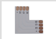
L 字型 RGB 基盤 品番：HBRGBPCL 基盤幅：SMD5050 サイズ
